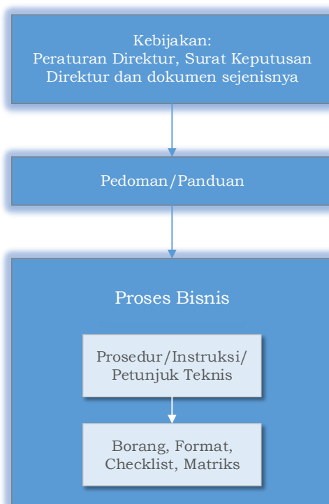
Gambar 2. Hierarki Dokumen
